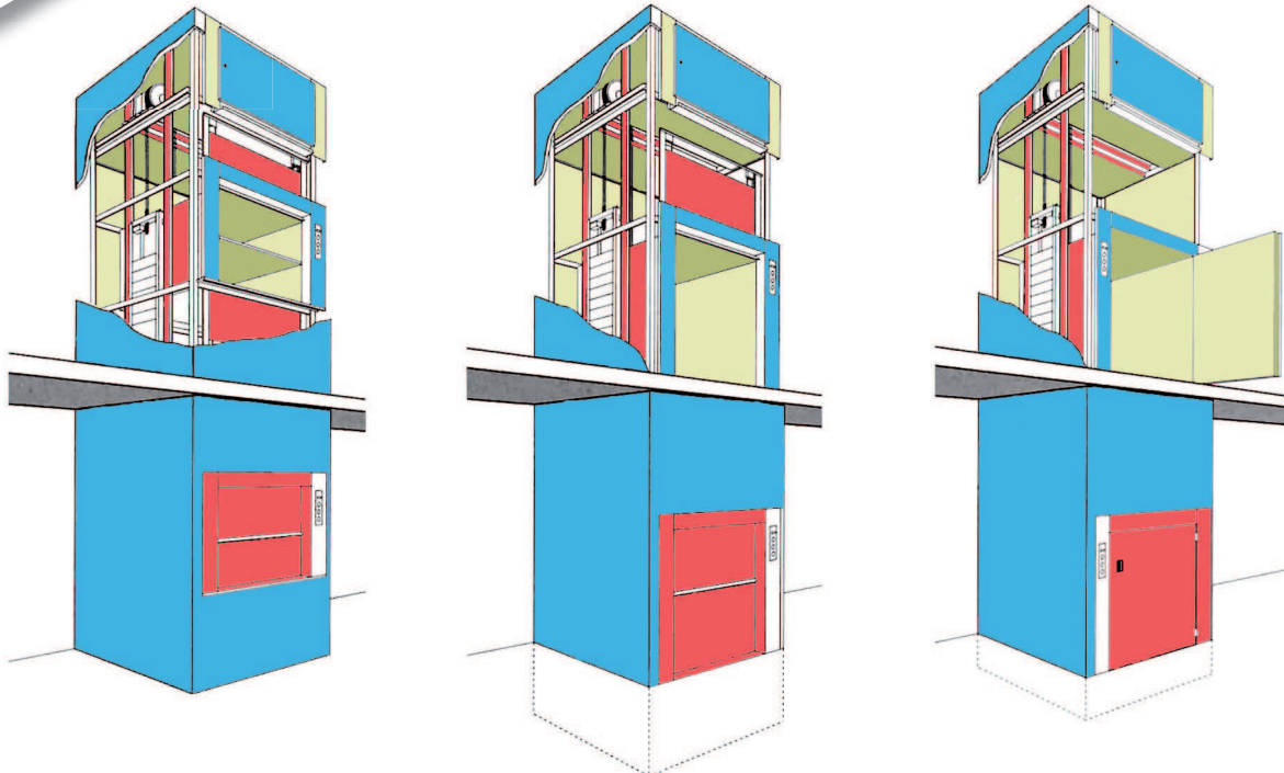
Portes à guillotines sur allèges
