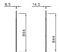
8,5/14,5mm lat. de acoplamento coupling panel jouis d'assemblage lat. de acoplamiento
