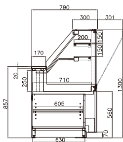
VELSNA - VDA neutra aberta opened dry ambient neutre ouvert neutra abierta
