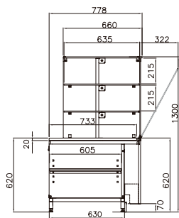
ELSTV torre de vidro tower glass tour vitrée torre de vidrio
