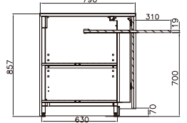
ELCXPMRTD caixa PMR c/ tampo PMR counter w/ top caisse PMR avec dessus caja PMR con tampo
