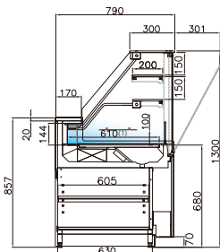
VELSVS - VDA 3M2 (1) ventilada superior upper ventilated ventilée supérieure ventilada superior
