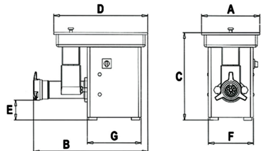
Tête de hachage entièrement en acier inox de haute qualité microfonderie.
