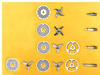
Systèmes de coupe disponibles : Simple (Enterprise), Double (Unger3) ou Quadruple (Unger5).
