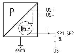
Connexion de charges à la sortie de commutation
