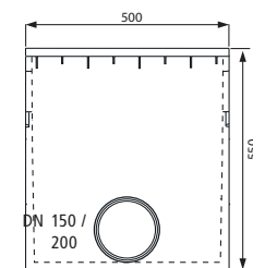
Boîte avaloir avec collecteur d'impuretés galvanisé
