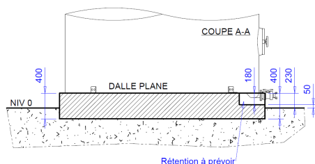
Plan de dalle pour cuve à fond plat :
