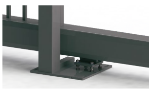
Chariot avant sur platine du poteau de guidage
