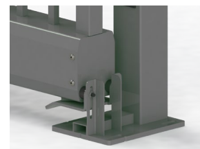
Lyre de réception basse avec butées
