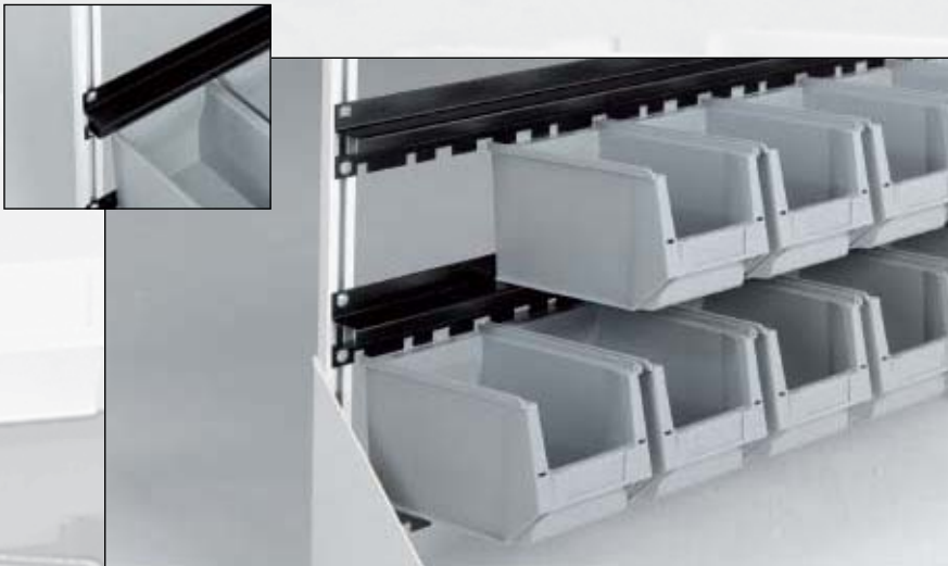
Dans nos profilés aluminium en C, les rails pour bacs Vario sont réglables. Chaque type de bac peut ainsi être suspendu.
