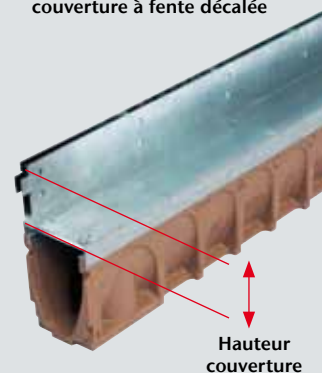
Caniveau Multidrain monté avec couverture à fente décalée
