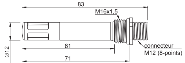
EE08 avec connecteur (Type D)
