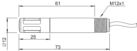
EE08 avec câble (Type E)
