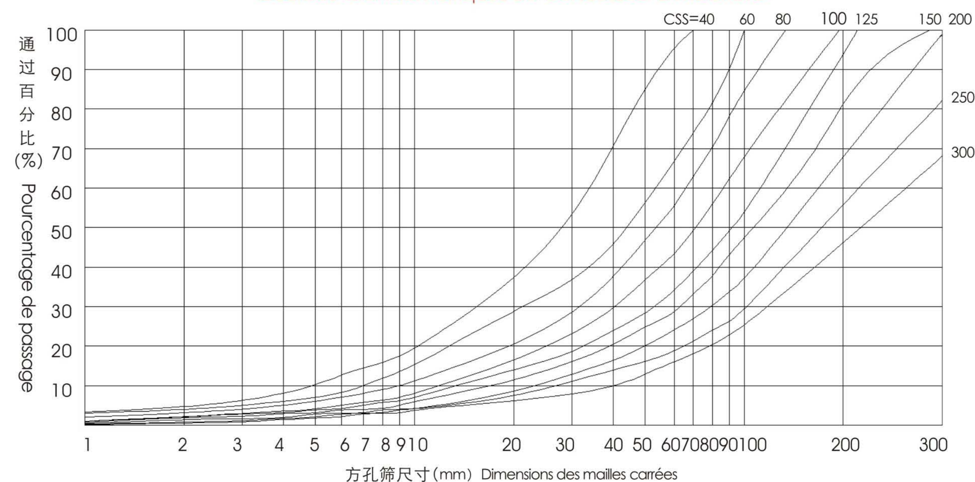
Courbes Granulométriques de Concasseur à Mâchoire
