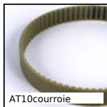
Courroie fermée, AT10 Polyuréthane armature acier
