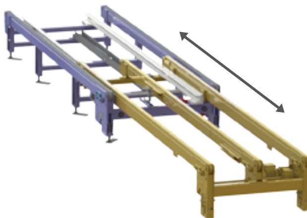
Convoyeur télescopique à allongement motorisé (passage de porte par exemple)
