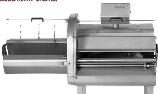
Slicco 650 en position de nettoyage avec protection panneau et porte devant ouverte
