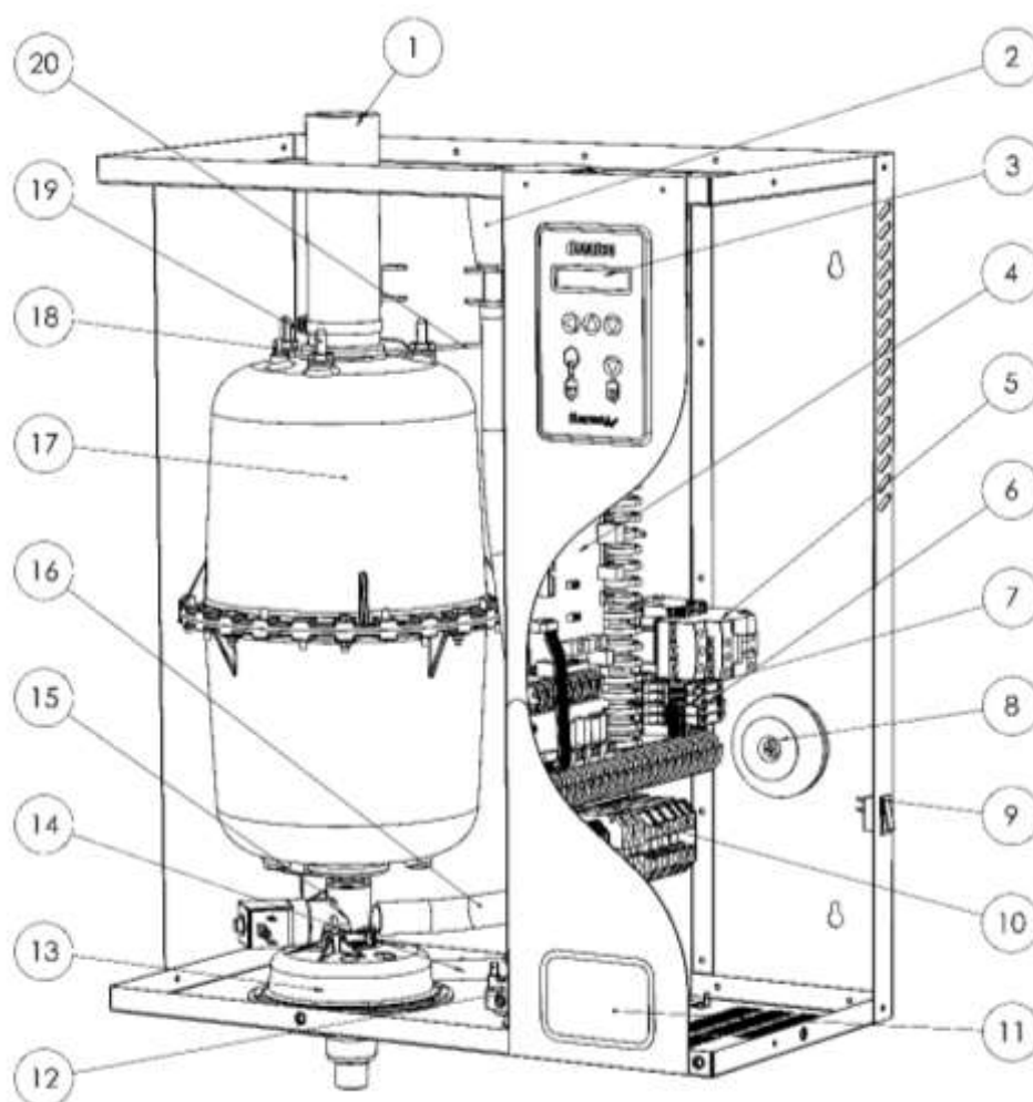
Fig. 2-3. Constitution de l'humidificateur
