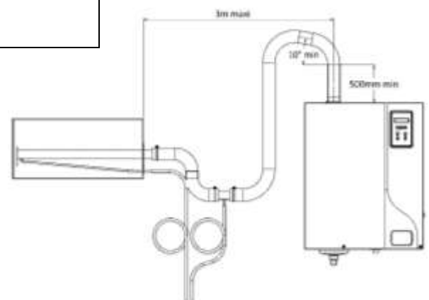
Fig. B 3-4. Purgé supplémentaire lorsque la vapeur est distribuée sous l'humidificateur
