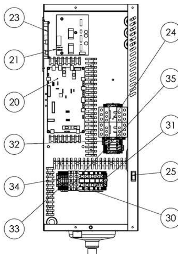
Fig. 7-4. Compartiment électrique
