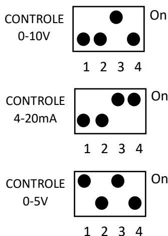
Configuration du Dip-Switch SW2 sur la carte principale
