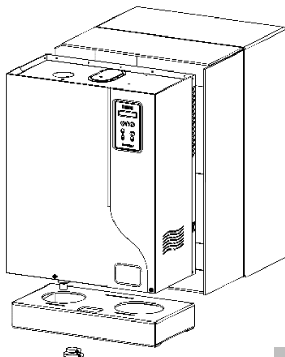
Fig. 2-1. Humidificateur
