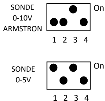
Configuration du Dip-Switch SW2 sur la carte principale
