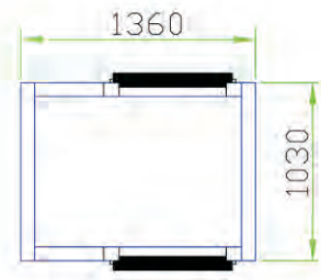
Vue en plan / Plan View
