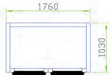
Vue en plan / Plan View
