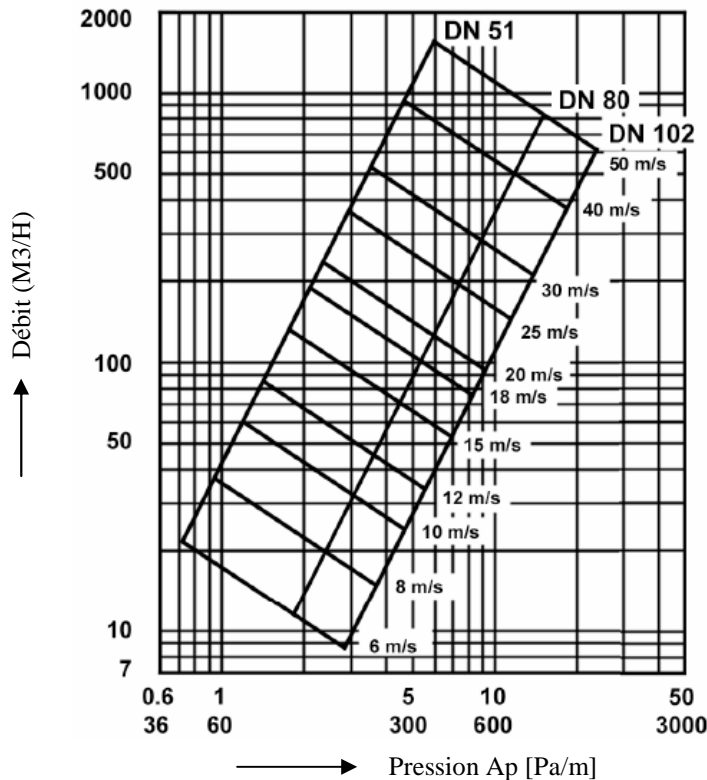
Type Master-PVC Flex flexible PVC très souple
