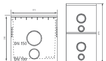
Boîte avaloir avec collecteur d'impuretés galvanisé
