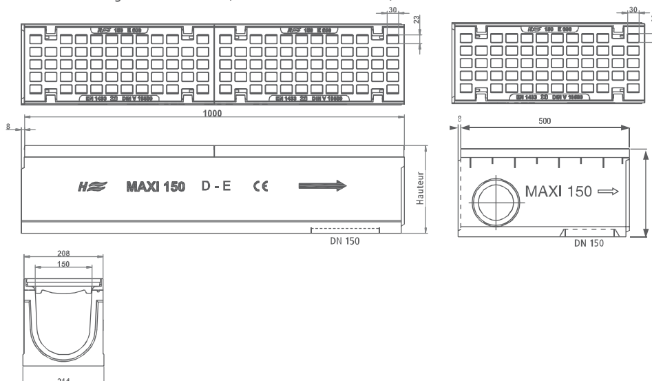
Boîte avaloir avec collecteur d'impuretés galvanisé
