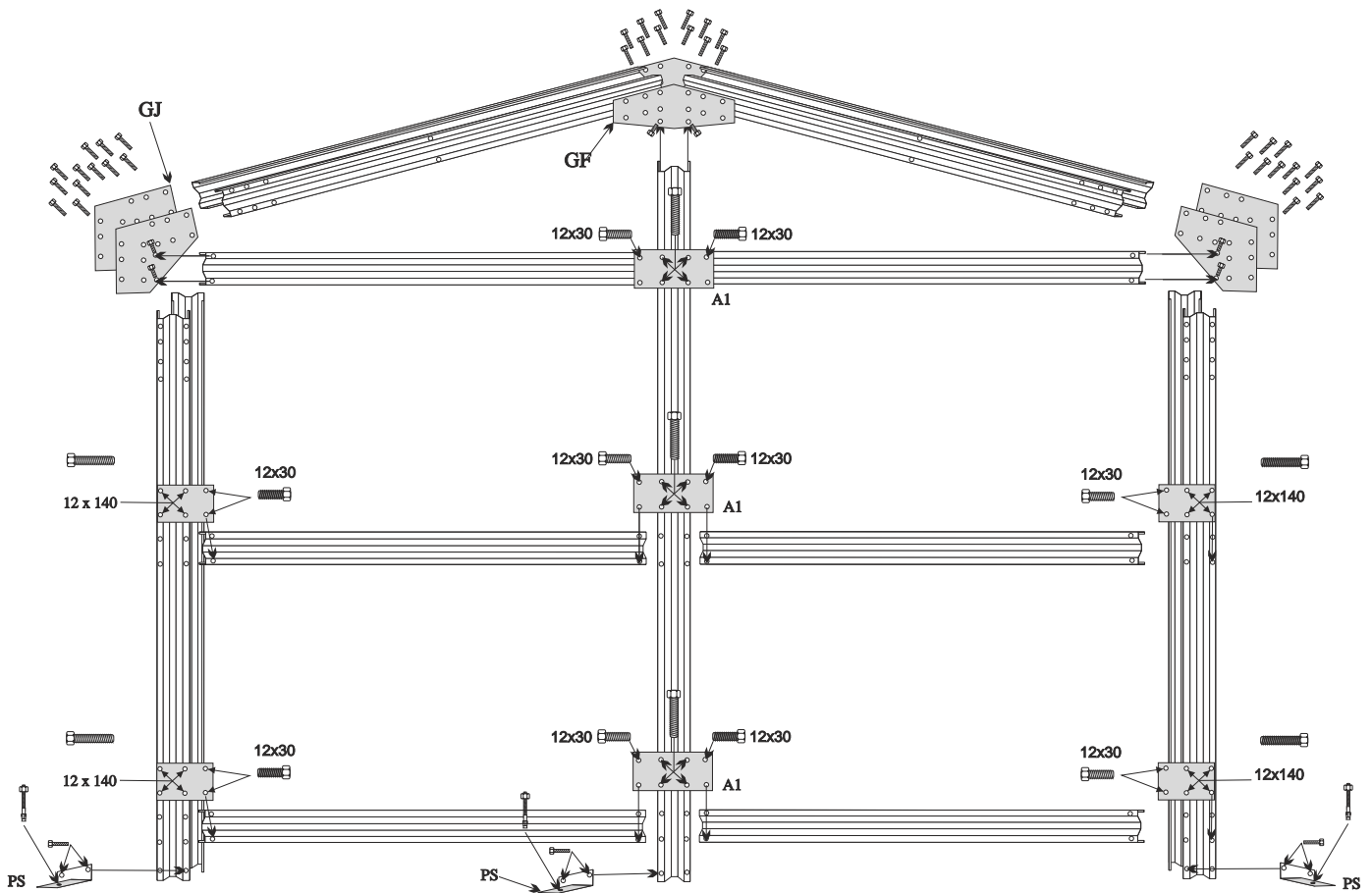
Montage ferme avec option ossature pignon
