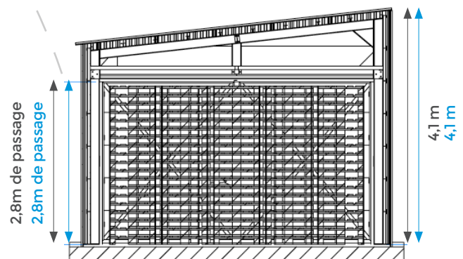
COUPE A
