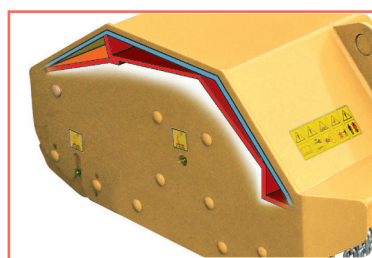
Protection interne pour le capot (séries SML et SML max)
