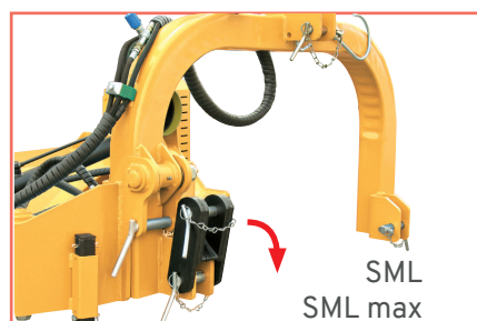
Attelage trois points avec dispositif de sécurité
