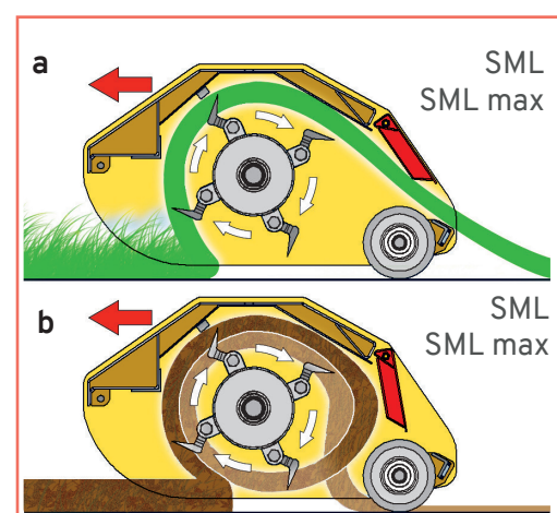
Position du capot pour le broyage de l'herbe (a) et pour le bois (b)
