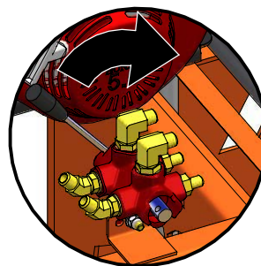
Vue A Sélecteur de valve
