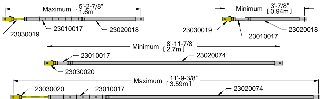
Figure C.25 Longueur d'ajustement des tendeurs
