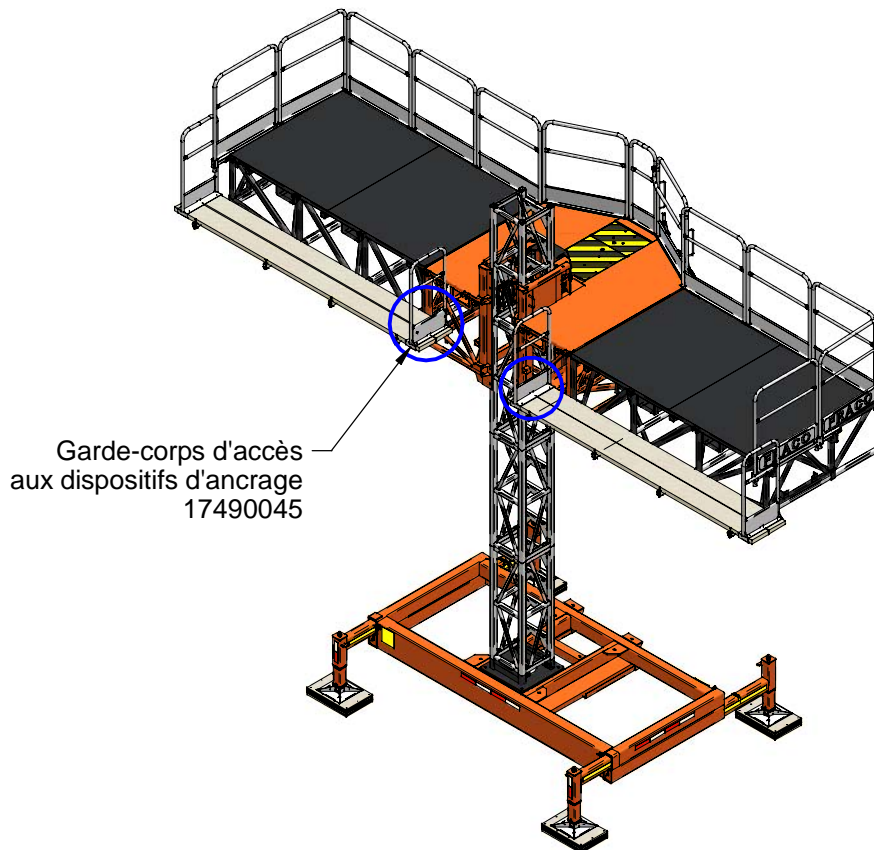
Figure E.35 Garde-corps d'accès
