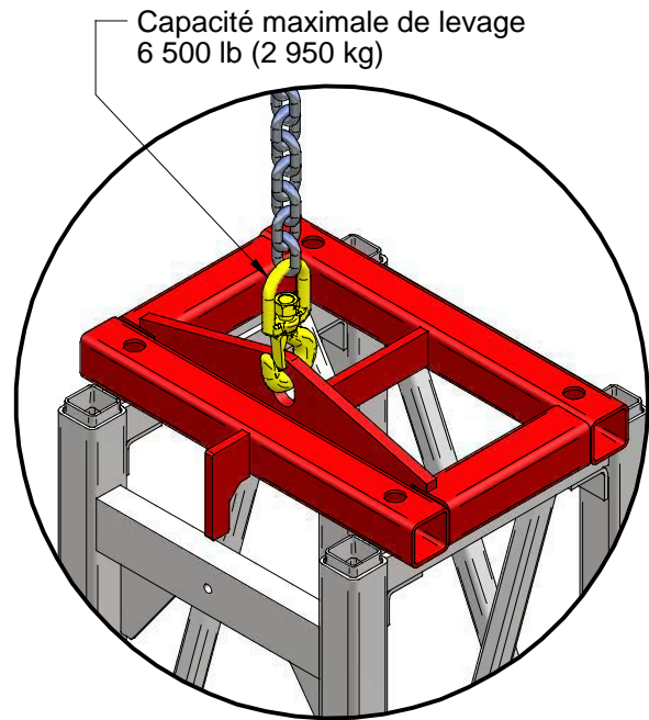
Figure C.2 Capacité maximale de levage
