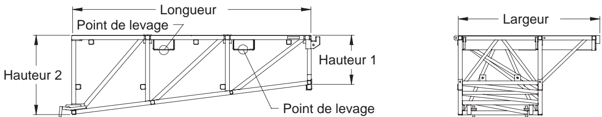
Figure D.2 Dimensions des sections de porte-à-faux effilées modulaires
