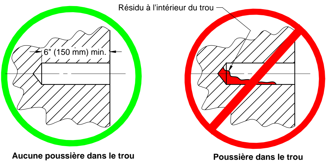
Figure C.54 Propreté dans le trou
