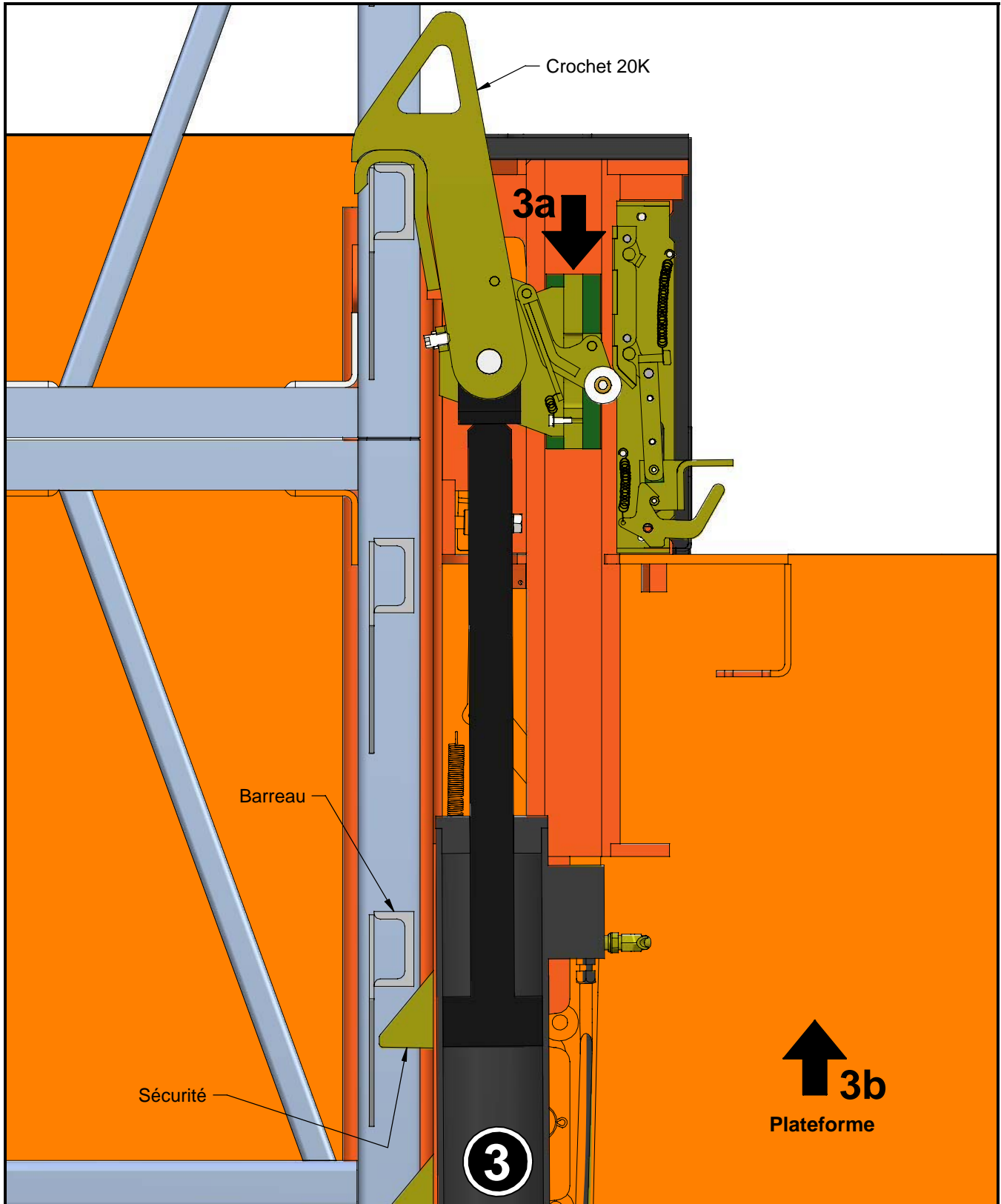
Figure A.4c Mécanisme en mouvement (Élévation)
