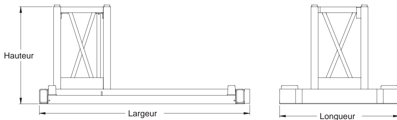
Figure B.2 Dimensions de la base au sol
