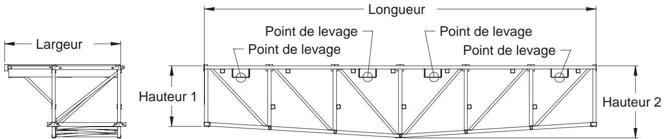
Figure D.5 Dimensions des sections de ponts modulaires
