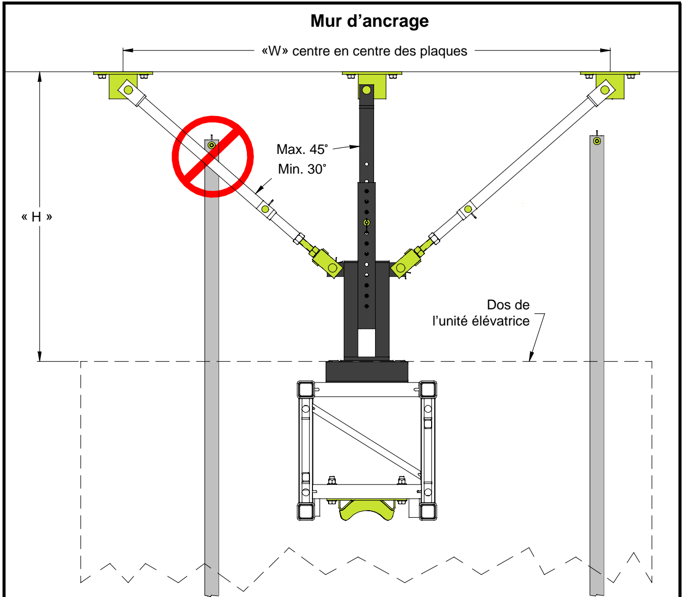
Figure C.27 Contraintes d'ouverture des tendeurs
