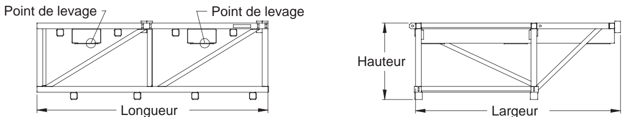
Figure D.1 Dimensions des sections de porte-à-faux modulaires
