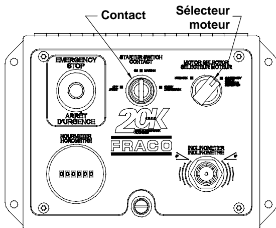
Boîtier de contrôle 20K
