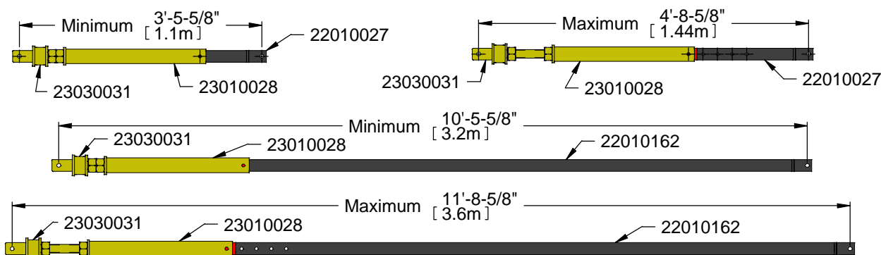
Figure C.26 Longueur d'ajustement des tendeurs renforcis
