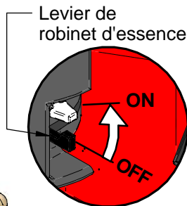
Vue K Levier de robinet d'essence
