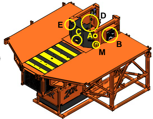
Pivot d'opération 20K
