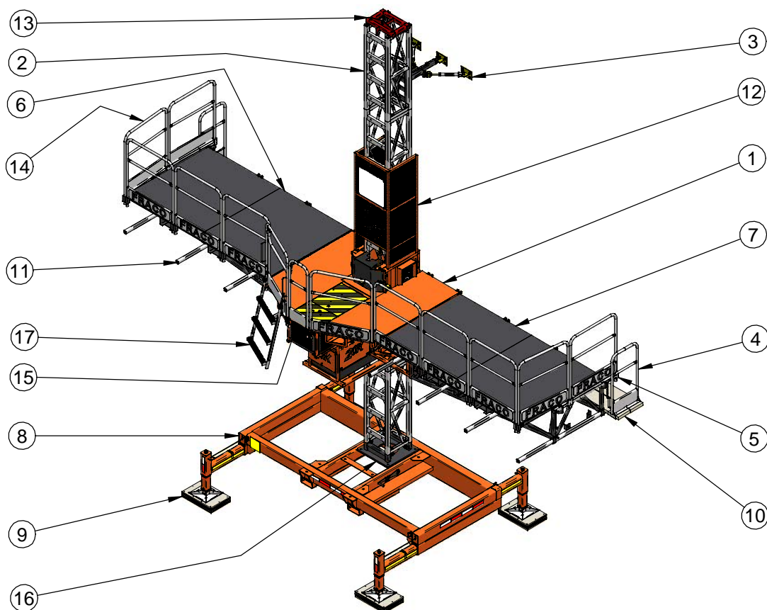
Figure A.2a Vue générale (mono-mât)
