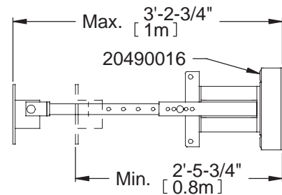
Figure C.21 Dimensions avec le petit dispositif d'ancrage
