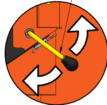
Vue D Pivot d'opération 20K (horaire, le cylindre ouvre) (anti-horaire, le cylindre ferme)
