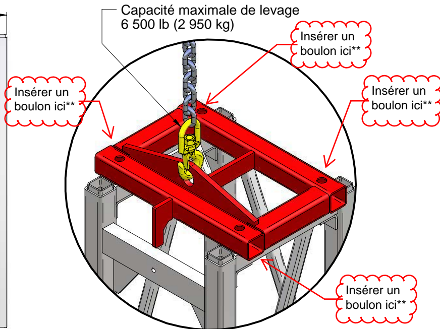
Figure C.2 Capacité maximale de levage
