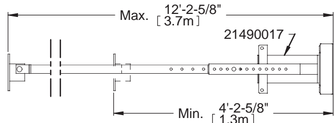
Figure C.22 Dimensions avec le grand dispositif d'ancrage
