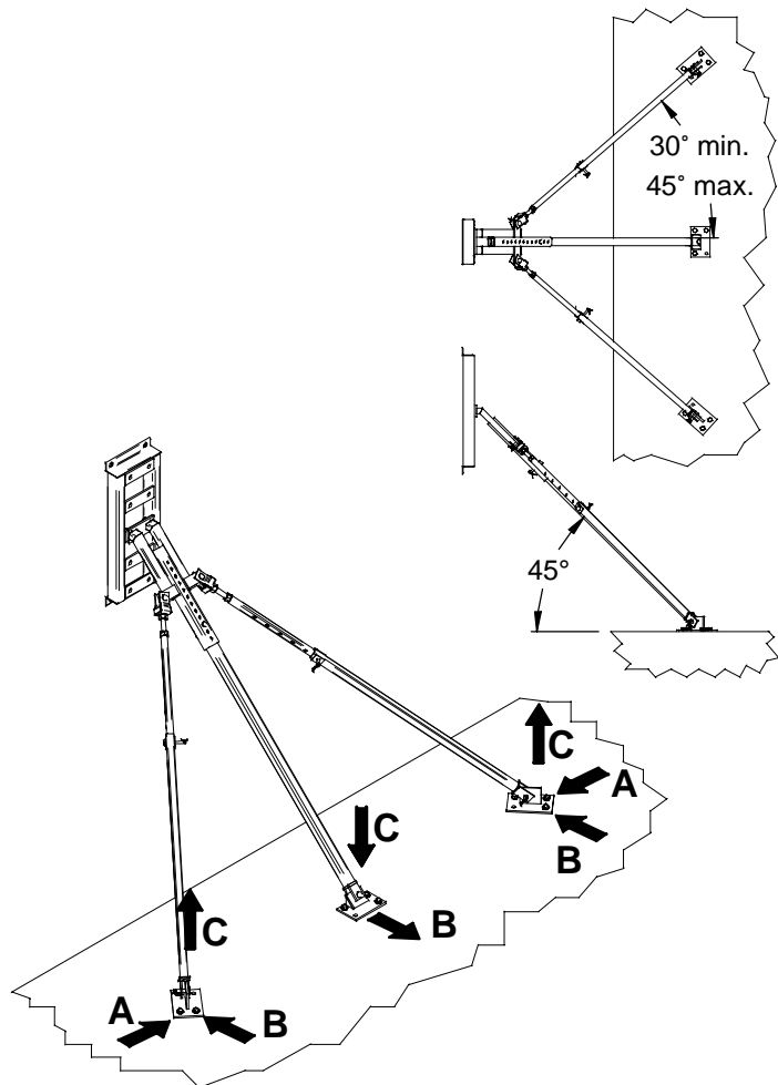
Figure C.8 Dispositif d'ancrage à trois (3) points en angle sur la dalle
