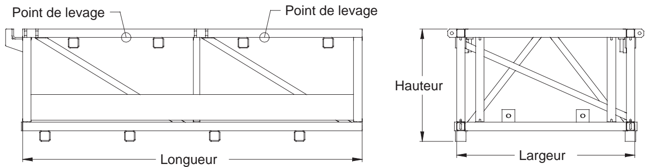
Figure D.3 Dimensions des sections de porte-à-faux non-modulaires
