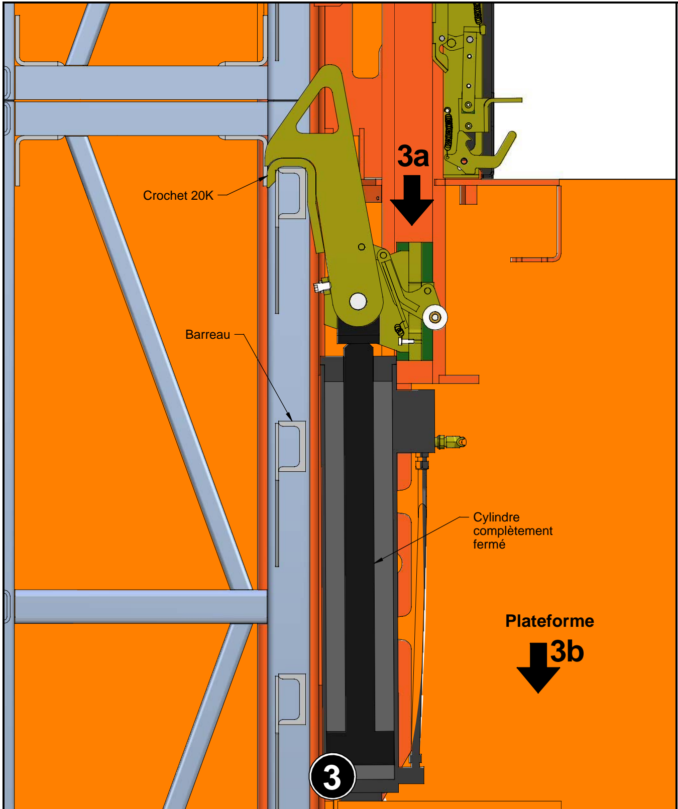
Figure A.4f Mécanisme en mouvement (Descente)
