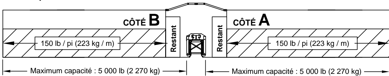
Figure A.3b Configurations (maçonnerie)
