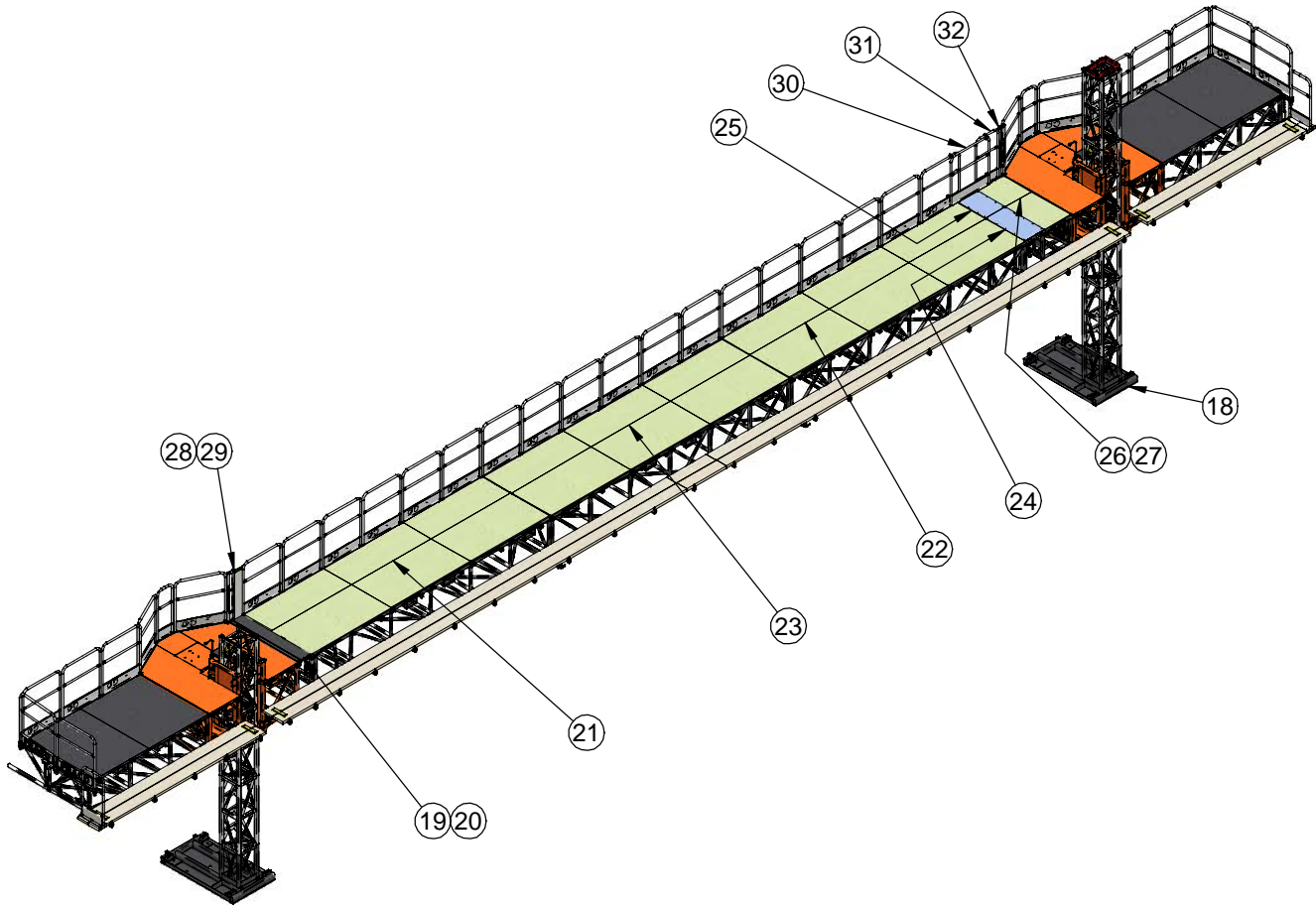
Figure A.2b Vue générale (double-mât)
