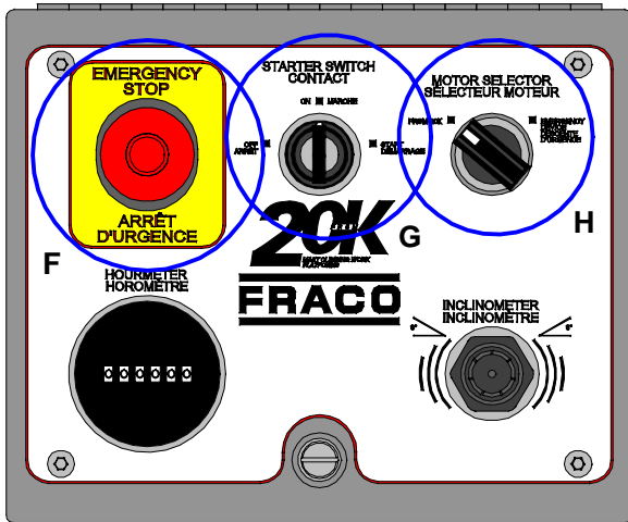
Vue B Boîtier de contrôle FRSM-20K
