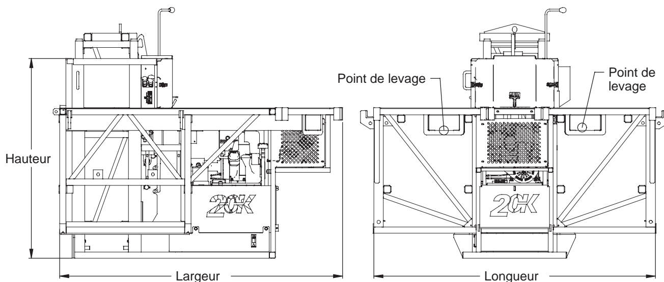
Figure B.1 Dimensions de l'unité élévatrice
