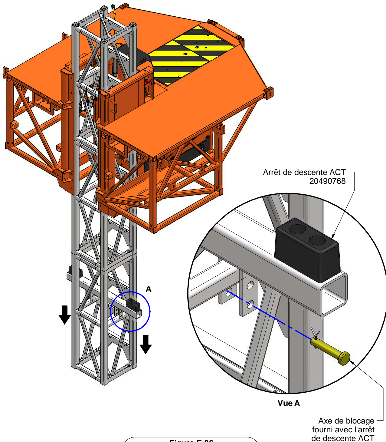
Figure E.36 Arrêt de descente ACT
