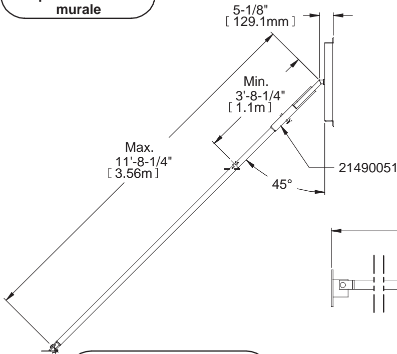
Figure C.20 Dimensions avec le dispositif d'ancrage en angle
