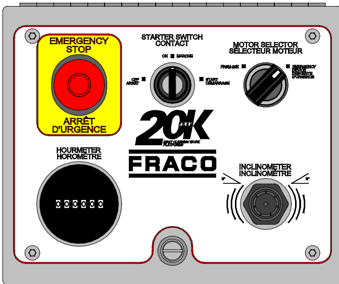
Vue B Boîtier de contrôle 20K
