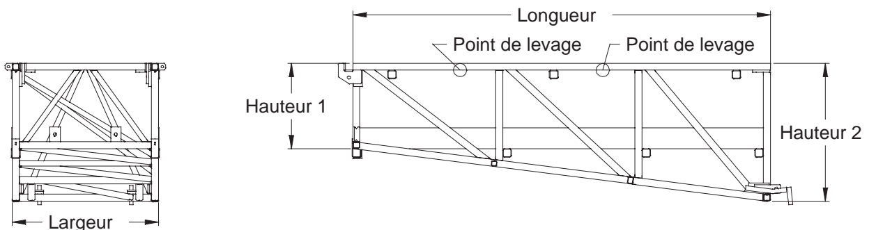
Figure D.4 Dimensions des sections de porte-à-faux effilées non-modulaires
