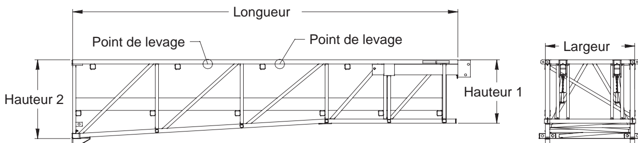
Figure D.7 Dimensions des sections de ponts non-modulaires
