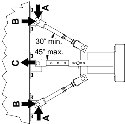
Figure C.6 Dispositif d'ancrage à trois (3) points en façade de ladalle
