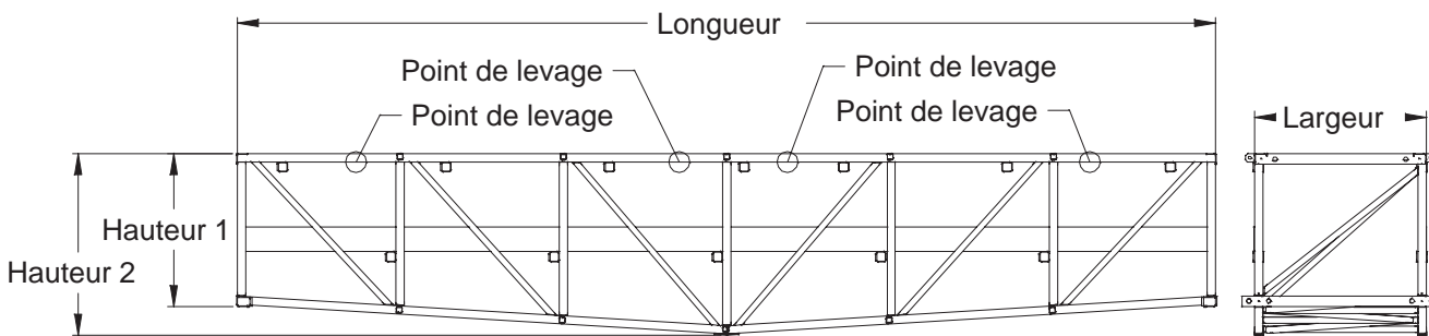
Figure D.7 Dimensions des sections de ponts non-modulaires
