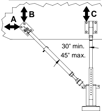
Figure C.7 Dispositif d'ancrage à deux (2) points en façade de la dalle
