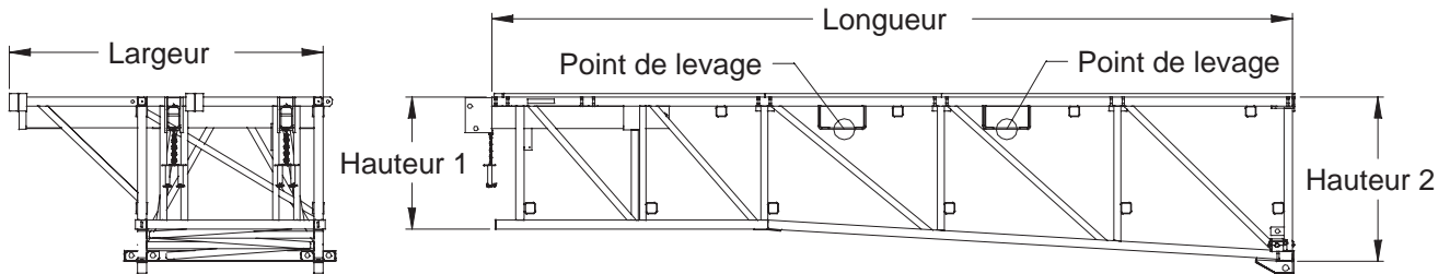
Figure D.5 Dimensions des sections de ponts modulaires
