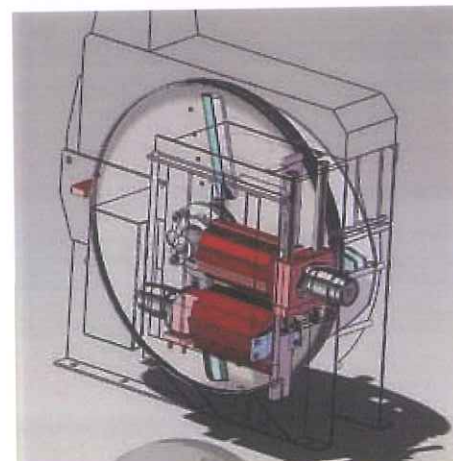
CIP 2200 - Dettaglio Gruppo rulli alimentatori
