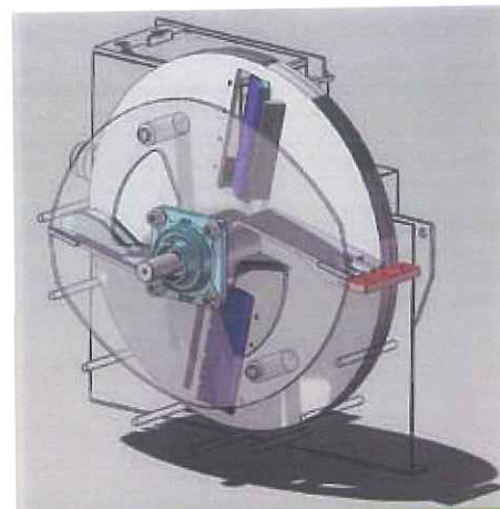
CIP 2200 - Dettaglio Sistema di raffinazione e calibratura
