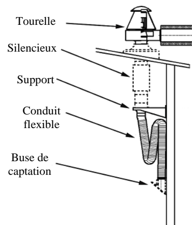
Unité d'aspiration simple avec ventilateur en toiture
