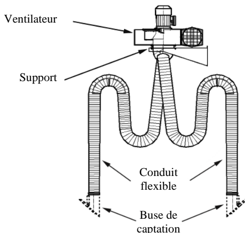
Unité d'aspiration double avec ventilateur sur support mural
