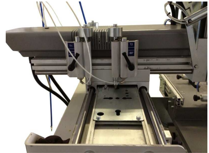
Palpeurs T1 et T2 pour la réalisation des usinages avec la table en position -90^\circ et +90^\circ
