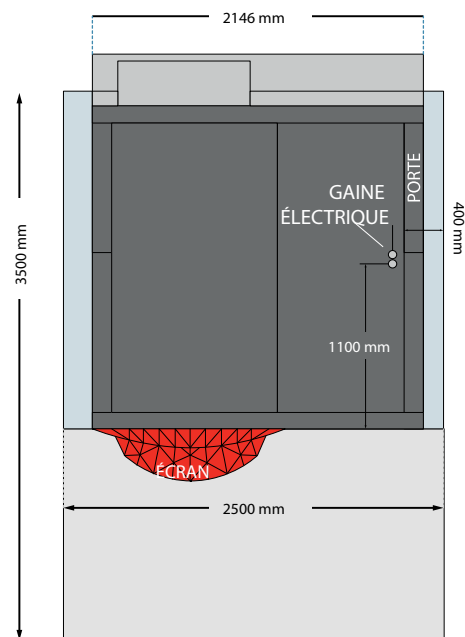
DESSUS - PORTE DROITE
