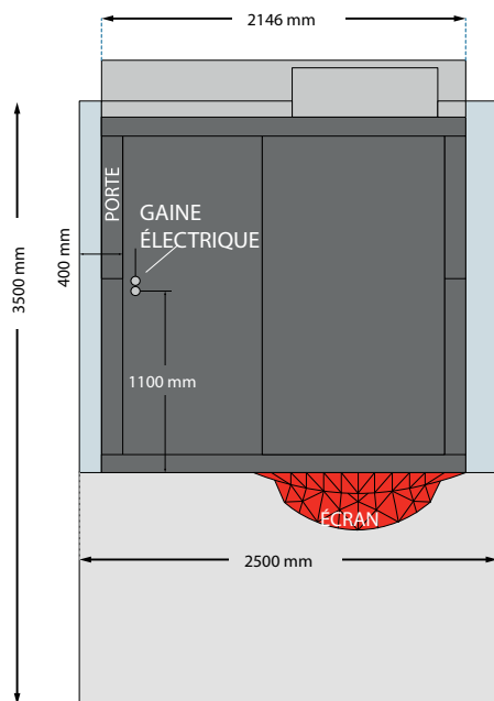
DESSUS - PORTE GAUCHE
