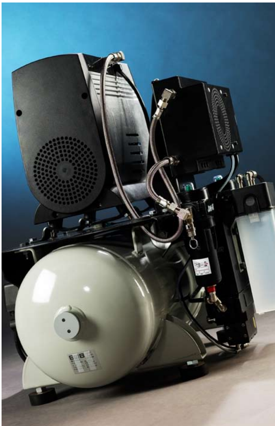
Modèle OF1201-25HBD2
