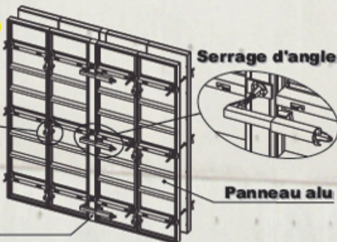
Lisse de compensation Largeur 5 ou 10 cm
