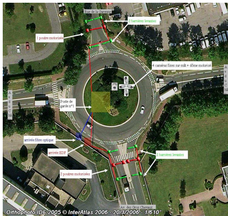
Synoptique vidéosurveillance
