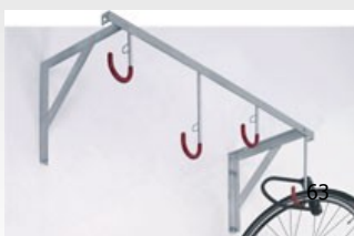
63 INDOOR-A et 64 INDOOR-D suspension murale collective (A) ou individuelle (D) option sécurisation du cadre (D) | wall-suspension, multi-space (A) or 1-space (D) with the option of frame padlocking (D)
